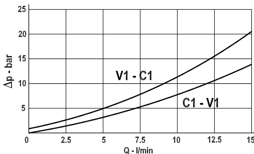
DIAGRAMMA PERDITE DI CARICO PRESSURE DROP CURVES
