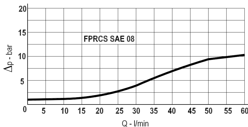
DIAGRAMMA PERDITE DI CARICO PRESSURE DROP CURVES
