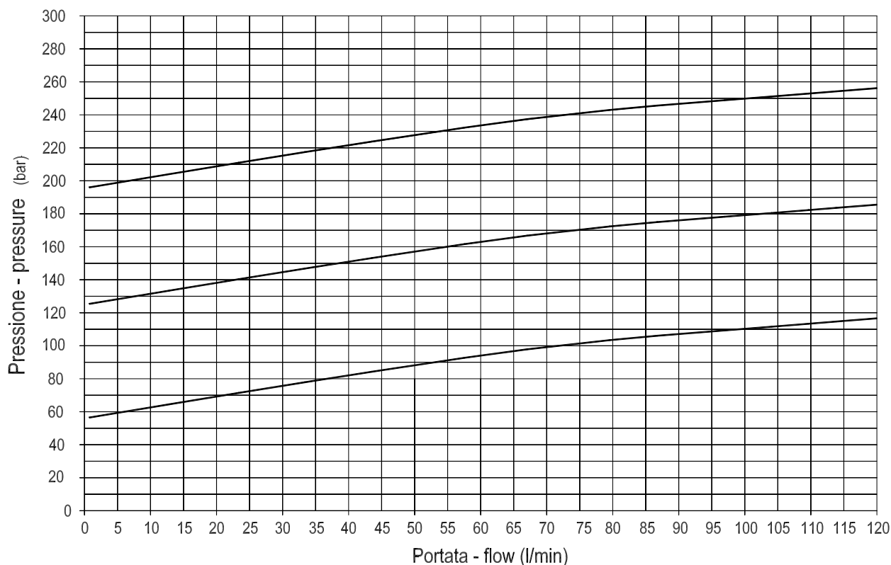
DIAGRAMMA PERDITE DI CARICO PRESSURE DROP CURVES
